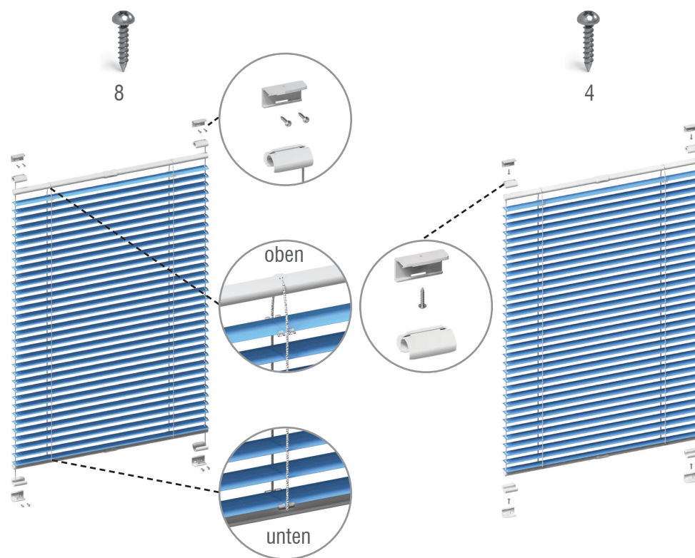
Abb. 3 - Rahmenmontage
